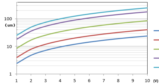
图 2 驱动频率为谐振频率时，驱动电压与光程差
