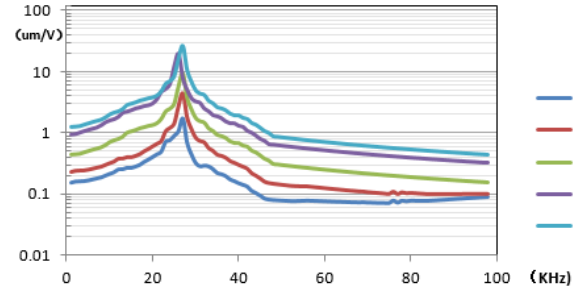
图 3 1HZ-100KHz 扫频时，驱动频率与光程差系数
